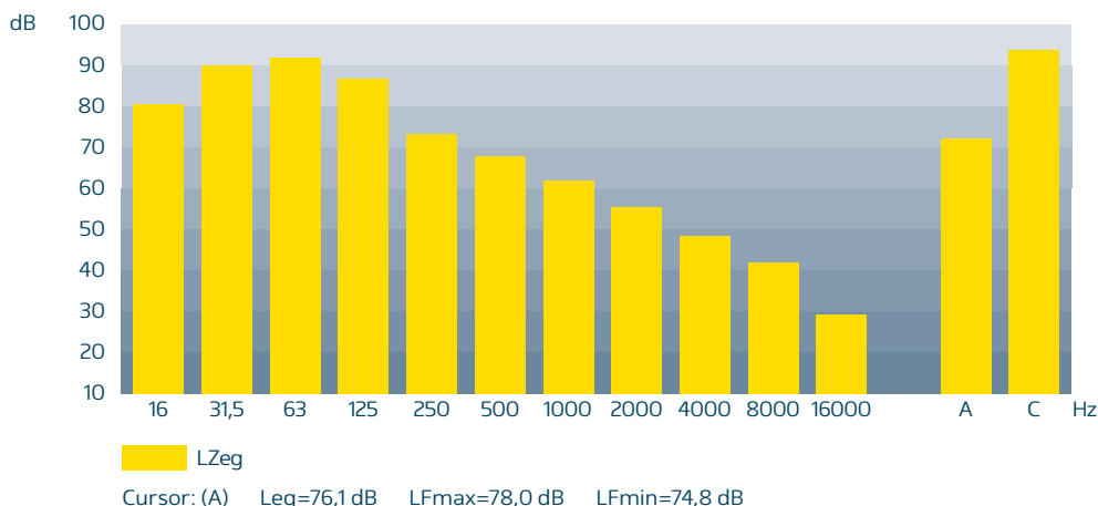
Figur 3 - Måling efter ombygning - Gennemsnit: 69,2 dB (A)
