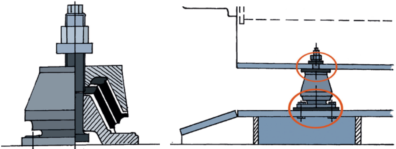
Figur 27 og 28 Svingningsdæmpere
