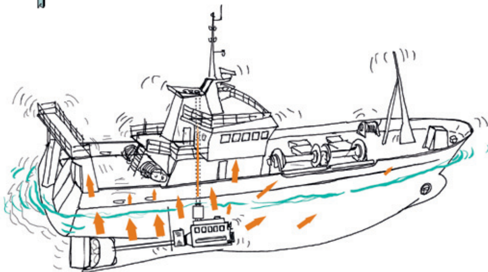
Figur 7 og 8 - Strukturbåren støj
